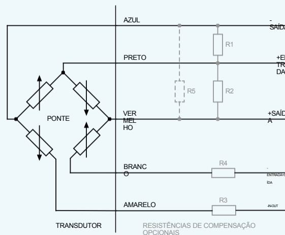
Esquema elétrico de um 7LHP com resistências de compensação
