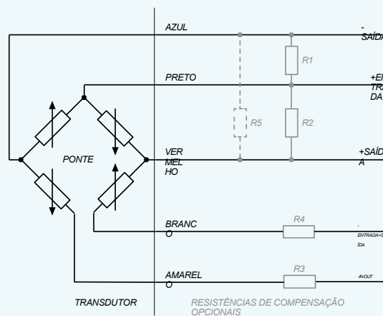
Esquema elétrico de um 7L com resistências de compensação
