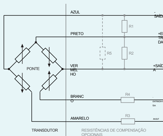
Esquema elétrico de um 9L com resistências de compensação
